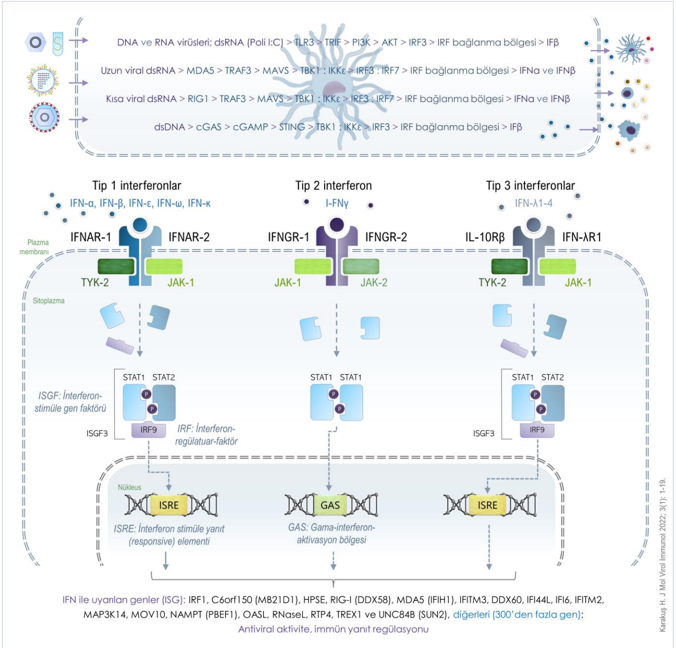
Şekil 1. İnterferon sinyal yollarına genel bakış. İnterferonların (IFN) üretimi, viral nükleik asitler gibi patojen kaynaklı moleküllerin hücre yüzeyine veya patern tanıma reseptörlerine (PRR) bağlanmasıyla başlar. Ortaya çıkan sinyal kaskadı, IFN'lerin transkripsiyonunu ve salgılanmasını aktive eder. Salgılanan IFN molekülleri aynı veya yakın hücrelerdeki ilişkili IFN reseptörlerine bağlanır. IFN'lerin reseptörlerine bağlanması, Janus tirozin kinazlar (JAK) ve tirozin kinaz (TYK) tarafından STAT1 ve/veya STAT2'nin fosforilasyonuna yol açan sinyal kaskadını aktive eder. Tip I ve III IFN'ler için, STAT1 ve STAT2 proteinleri IRF9 ile kompleks yapar ve IFN ile uyarılan yanıt ( responsive ) elemanlarına (ISRE) bağlanırlar ve sonraki basamakta IFN ile uyarılan genler (ISG) aktive edilir. Tip II IFN'ler ise fosforile edilmiş STAT1 dimerlerinin gama ile aktive olan bölge (GAS) elementlerine bağlanmasını uyarır ve süreç ISG'lerin uyarılması ile devam eder. Sonraki aşamalarda tip I, tip II veya tip III IFN'ler ile aktive edilen ISG'ler ( 300'den fazla gen ) enfekte hücrelerdeki geniş kapsamlı veya belirli virüsler için spesifik antiviral etkilere doğrudan aracılık edebilir veya doğuştan gelen ve adaptif bağışıklık tepkilerini indükleyebilir ( pozitif regülasyon ) veya inflamasyonun baskılanması ( negatif regülasyon ) gibi farklı mekanizmalarla immün yanıtı düzenleyebilir [4,16,18,27,32-35]. (Çizim: Hasan Karakuş, Fatih Şahiner)
